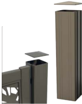
SCELLEMENT 400 MM 188 x 188 mm Rainuré . Alu à sceller
